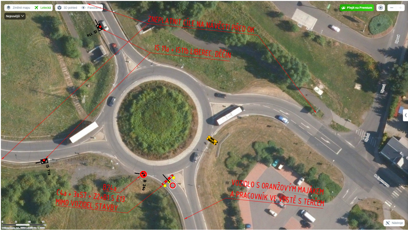
OKRUŽNÍ KŘIŽOVATKA I/9 A ULICE B. EGERMANNA
